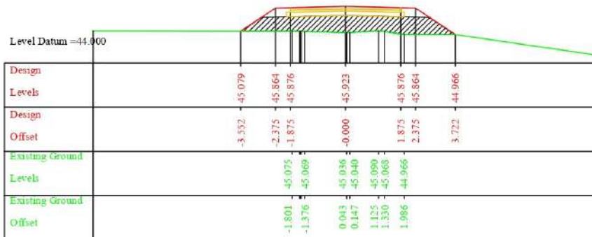
Chainage =300.000
