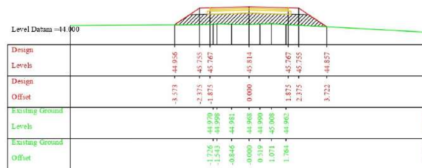
Chainage =330.000
