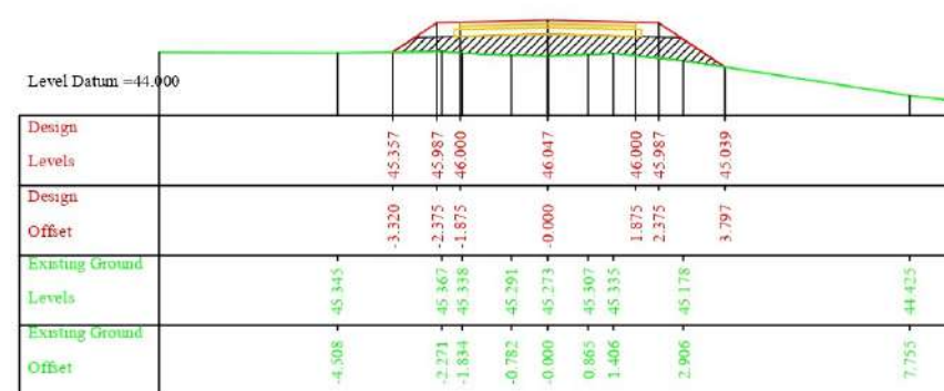
Chainage =270.000
