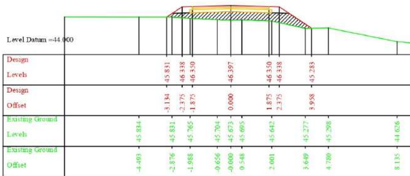
Chainage =180.000
