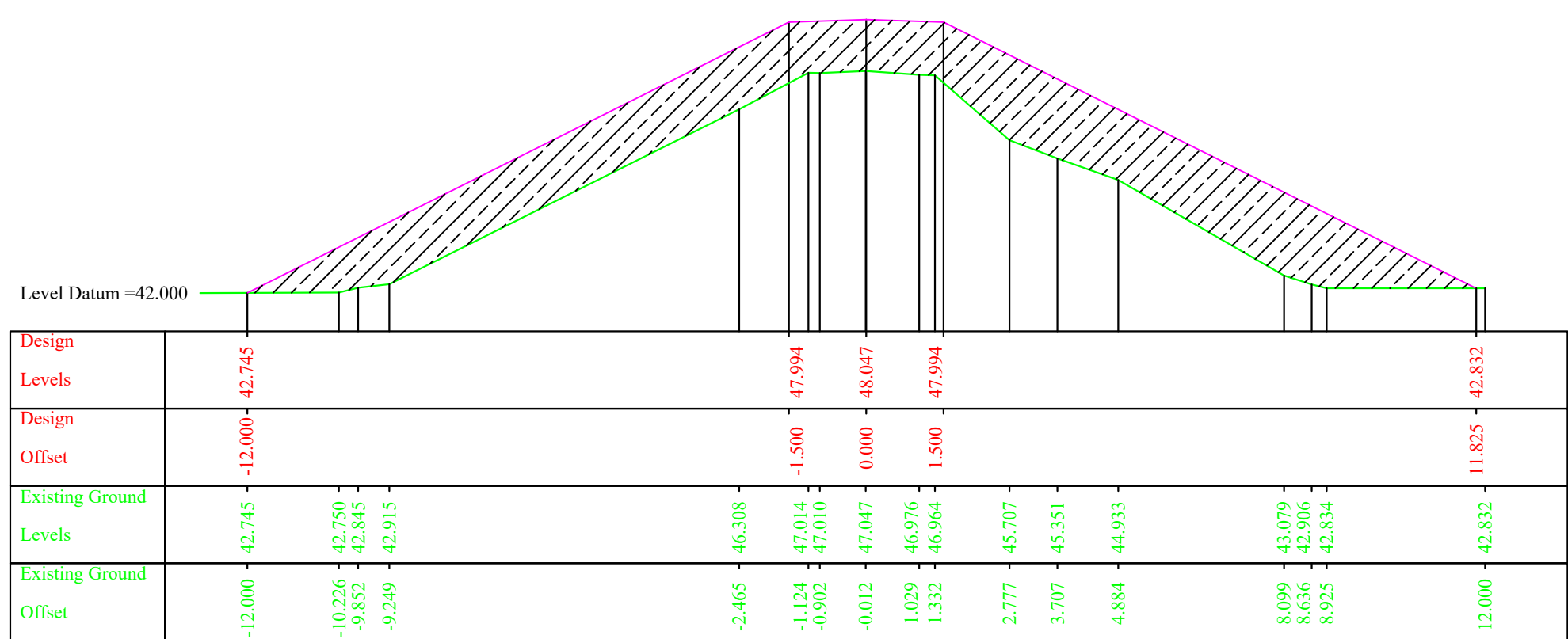
Chainage =780.000
